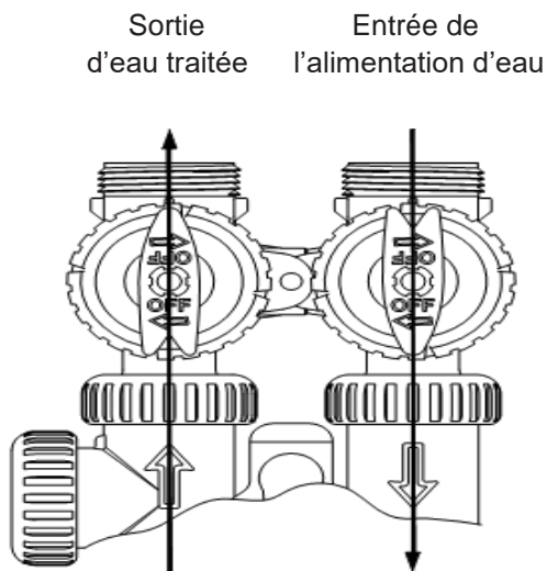
Figure 1 Opération normale
