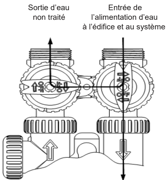
Figure 3 Mode diagnostique
